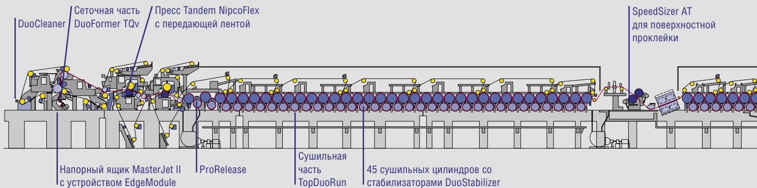
Компоновка БДМ-10.
